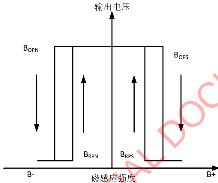
图 6. 磁场特性图
